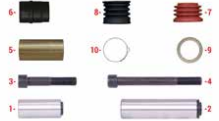
Kısa Pim 34x80 Uzun Pim 36x145
